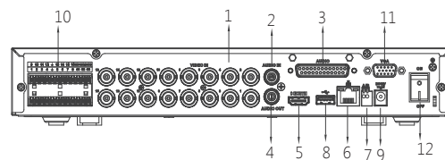
DH-XVR7116HE-4KL-X
